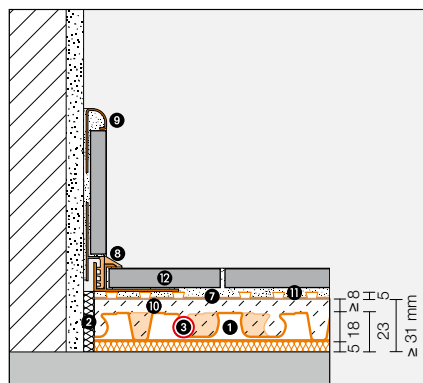
Estrutura de Schlüter®-BEKOTEC-EN 18 FTS com tubo de climatização 12 x 1,5 mm
