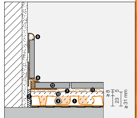
Montagem Schlüter®-BEKOTEC-EN 23 F com tubagem de climatização 14 x 2 mm
