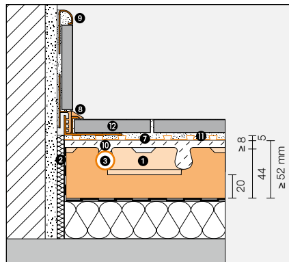
Montagem Schlüter®-BEKOTEC-EN/P ou -EN/PF com tubagem de climatização 16 x 2 mm
