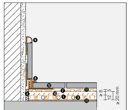
Estrutura de Schlüter®-BEKOTEC-EN 12 FK com tubo de climatização 10 x 1,3 mm
