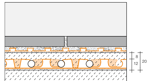
Estrutura com Schlüter®-BEKOTEC-EN 12 FK com tubo de climatização 10 x 1,3 mm Piso cerâmico climatizado de camada fina sobre betonilha existente
